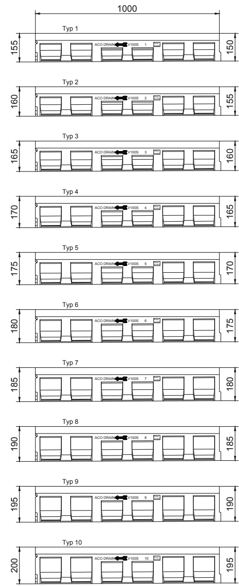
Улеи с вграден наклон 0.5%, дължина L=1m
