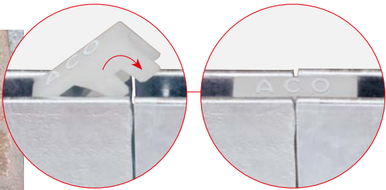
Използване на слот конектор за приеждаване на две решетки в права линия (при решетки от поцинкована или неръждаема стомана).
